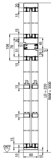
Вертикален разрез на стоманена врата с лофт дизайн, 2 крило, със странични части и оберлихт
