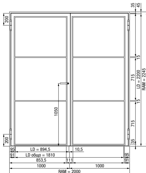
Стоманена врата с лофт дизайн, 2 крила
