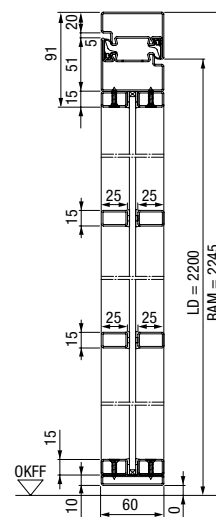
Вертикален разрез на стоманена врата с лофт дизайн, 1 крило
