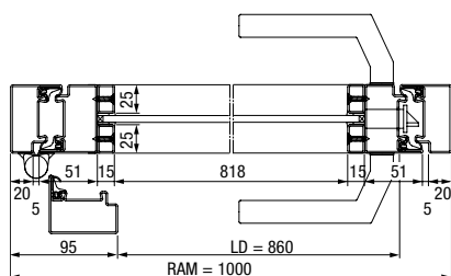
Хоризонтален разрез на стоманена врата с лофт дизайн, 1 крило
