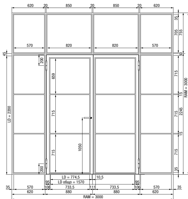
Стоманена врата с лофт дизайн, 2 крила, със странични части и оберлихт
