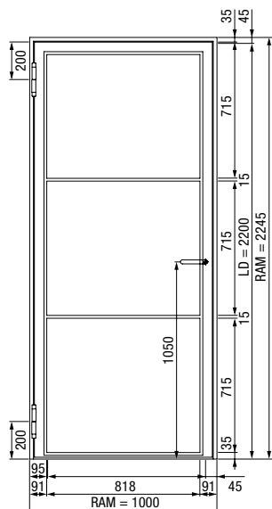
Стоманена врата с лофт дизайн, 1 крило
