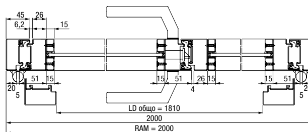
Хоризонтален разрез на стоманена врата с лофт дизайн, 2 крила
