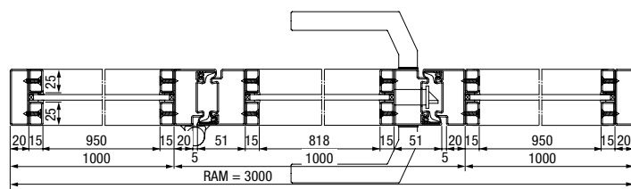
Хоризонтален разрез на стоманена врата с лофт дизайн, 1 крило, със странични части и оберлихт
