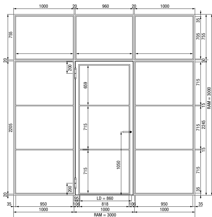
Стоманена врата с лофт дизайн, 1 крило, със странични части и оберлихт
