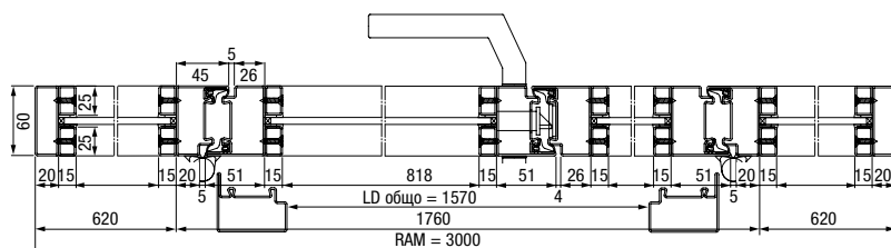
Хоризонтален разрез на стоманена врата с лофт дизайн, 2 крила, със странични части и оберлихт
